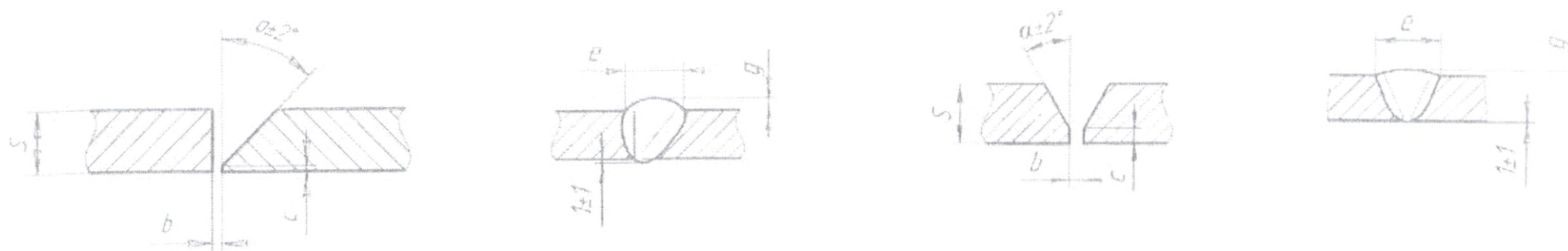
ИНСТРУКТИВНЫЕ ЭЛЕМЕНТЫ СОЕДИНЕНИЯ СВАРНОГО ШВА С17 ГОСТ 5264-80
